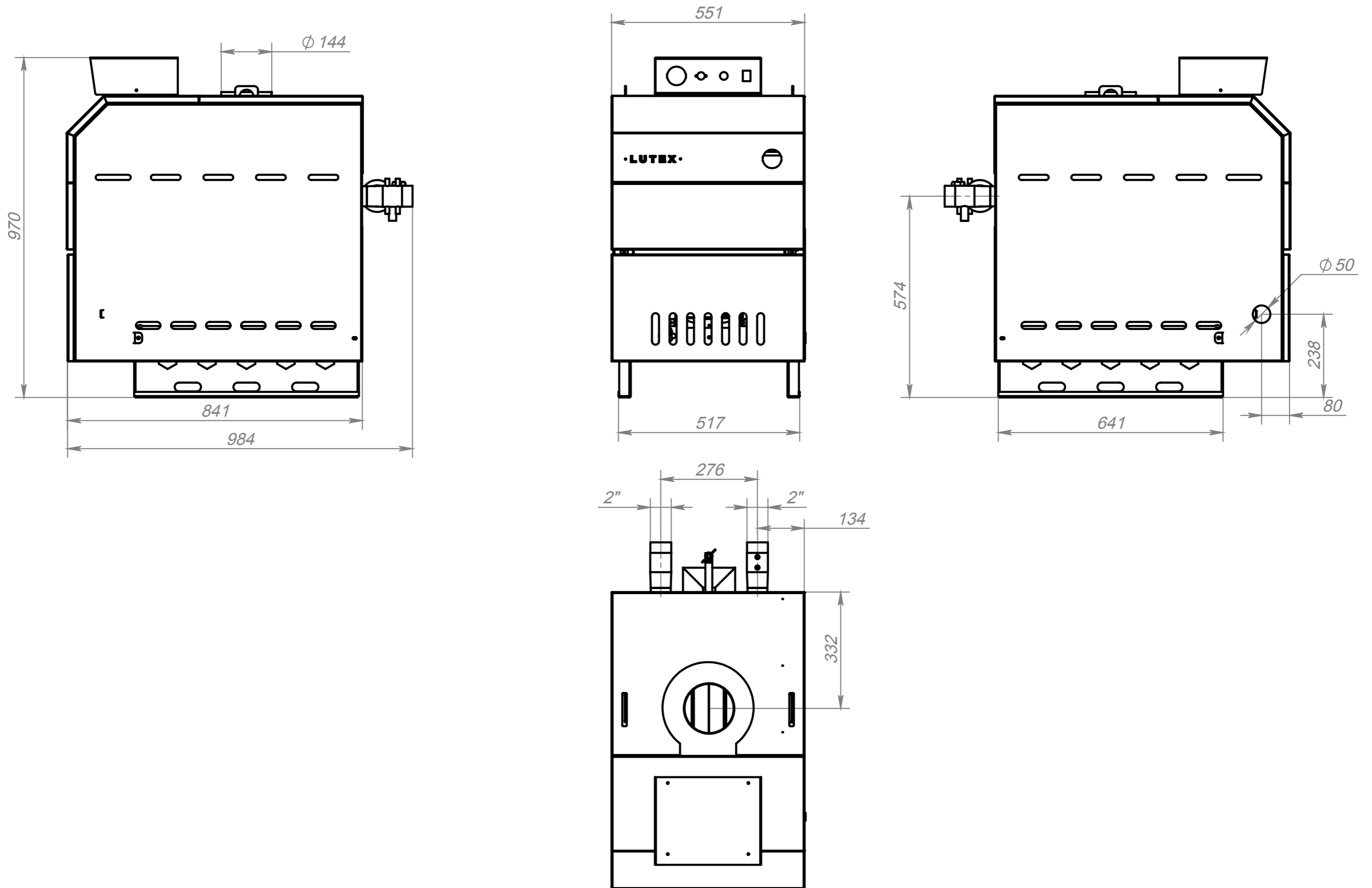
Габаритно-присоединительные размеры котла AR-S40
